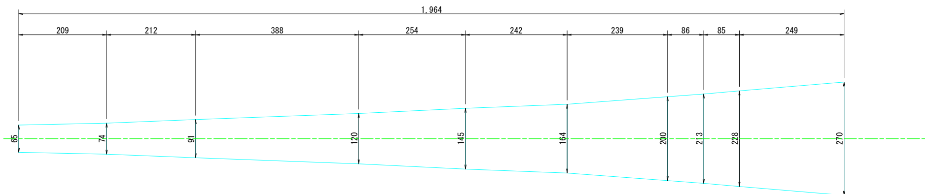
音道 広がり図 S=1/5
